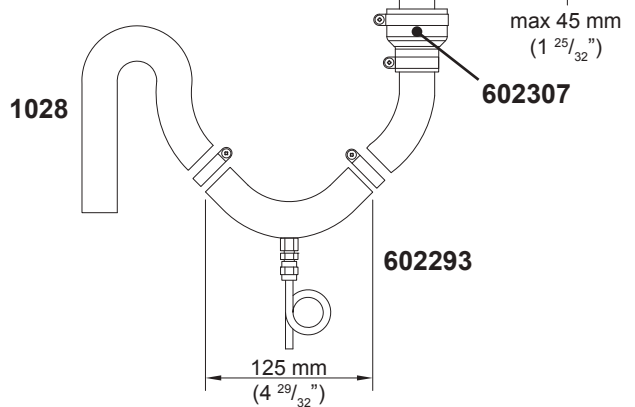
Installatie van de afsluitbare dakuitlaat 2466 . Het installatie gat is \varnothing 50 mm en de gaten van de schroeven 4 x 6 mm.
