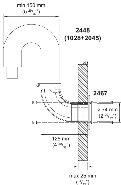
Sidegjennomføring 2467 er utført. Utskjæringen for installasjonen er \varnothing 50 mm og skruehullene er 4 \times \varnothing 6 mm
