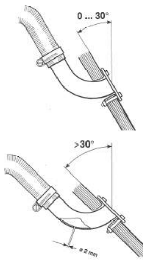
Installation à l'arrière du bateau
