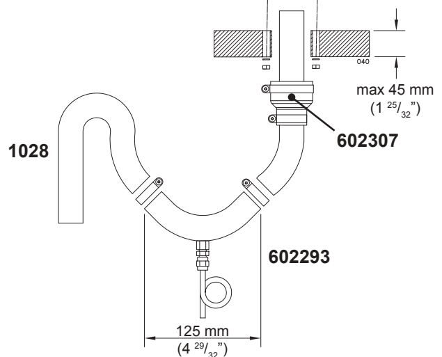
Установка закрываемого ввода для палубы 2466 . Монтажное отверстие - \varnothing 50 мм, отверстия для винтов - 4 x \varnothing 6 мм.
