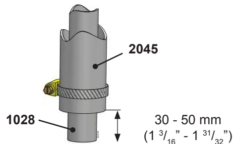
Putkien pituusero
