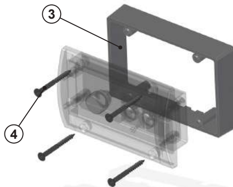
Vid ytinstallering av styrpanelen används halsen/kanten (3). I paketet medkommer 4 st festsättningskruvar, 3,5 x 40 mm (svart) TX 10 (4).
