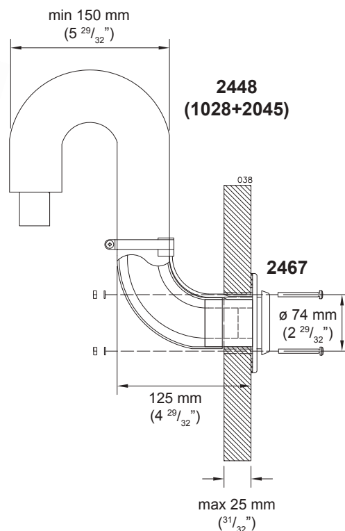
2467 sidogenomföring installerad. Installeringsutskärningen är Ø 50 mm och skruvhålen är 4 x Ø 6 mm
