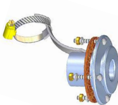
Rumpfdurchführung 2467
