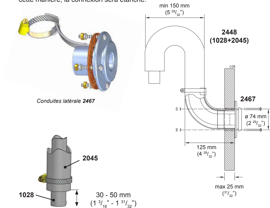
Différence de longueurs des tuyaux
