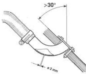
Installasjon på akterside
