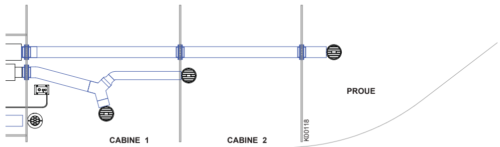
Dans les appareils 22 GB et 30 GB, c'est le tuyau supérieur qui est plus chaud.
