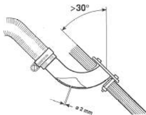
Установка на корме
