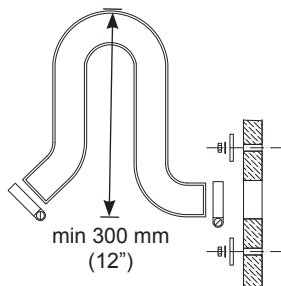
Cou de cygne
